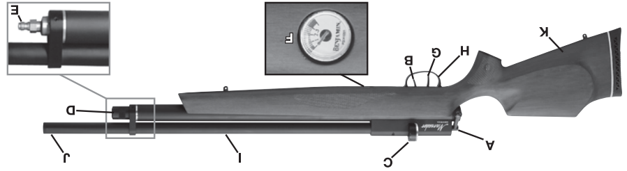
A. Cerrojo B. Seguridad C. Pinza D. Tapón protector del nipple de llenado E. Niple de llenado F. Medidor de presión G. Gatillo H. Guardamonte I. Carñón J. Boca K. Culata
